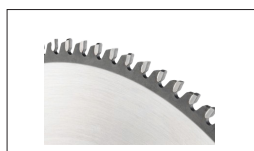
Réf : 10031 Lame carbure 355 x 2,6 x 25,4 mm – 90 dents
