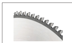
Réf : 10032 Lame carbure 355 x 2,6 x 25,4 mm – 80 dents
