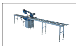
Réf : 2017C / 2020 Table d'amenage
