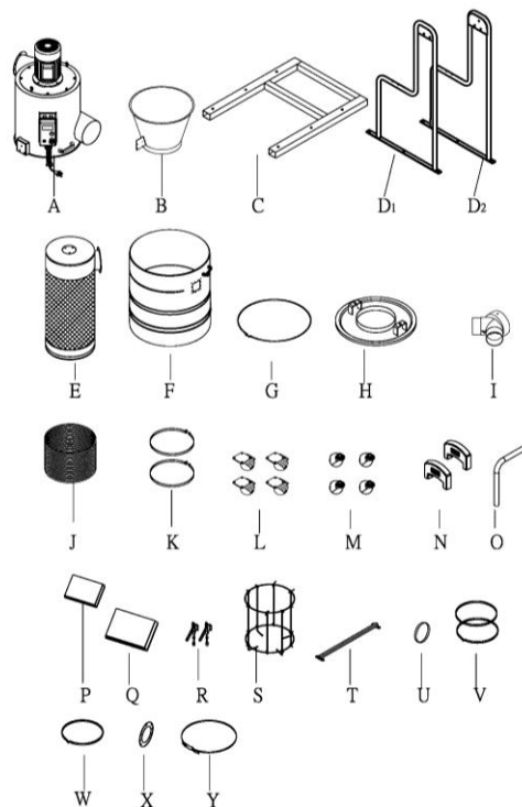
Figure 1 : contenu du carton principal (pas à l'échelle)
