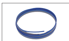
Réf : « Selon Denture » Ruban 5200 x 34 x 1.1 mm
